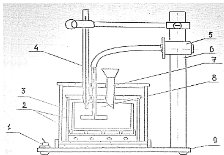
Рис. 1. Схема калориметра:
